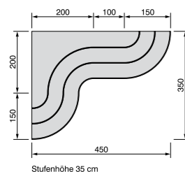
Stufenhöhe 35 cm
