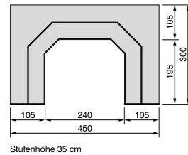
Stufenhöhe 35 cm
