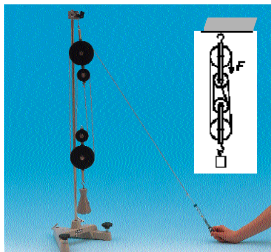
Esperimento con sistema di carrucole (342 28)
