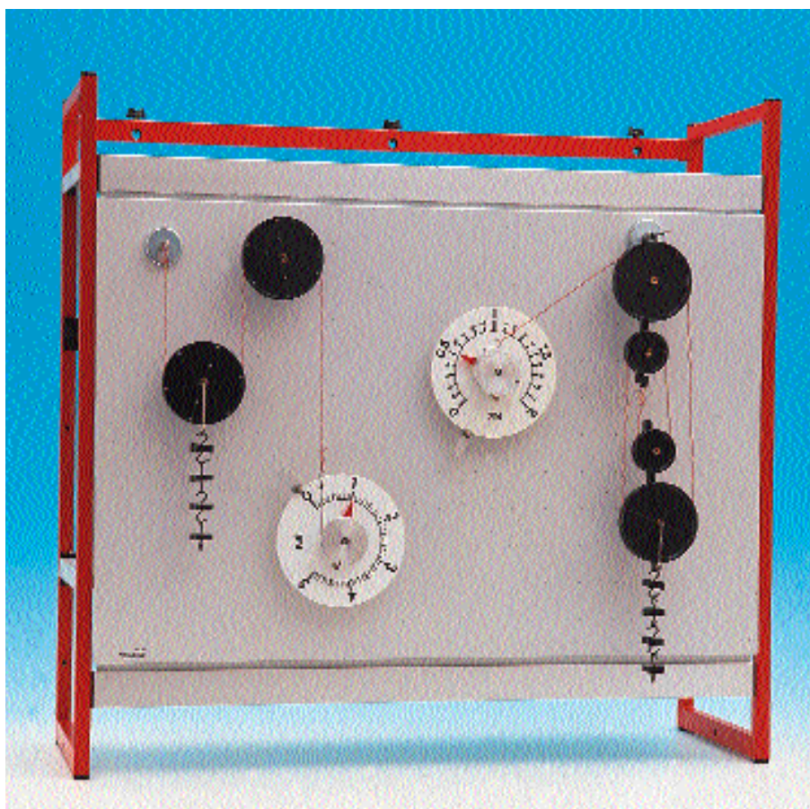
Carrucola fissa, carrucola mobile e sistema di carrucole come macchine semplici su tavola ad aderenza magnetica
